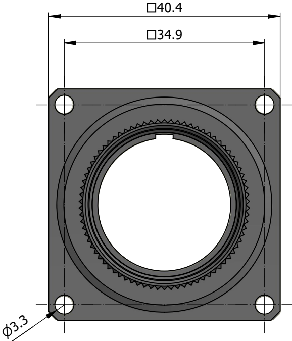
1) Shell Dimensions 1)
