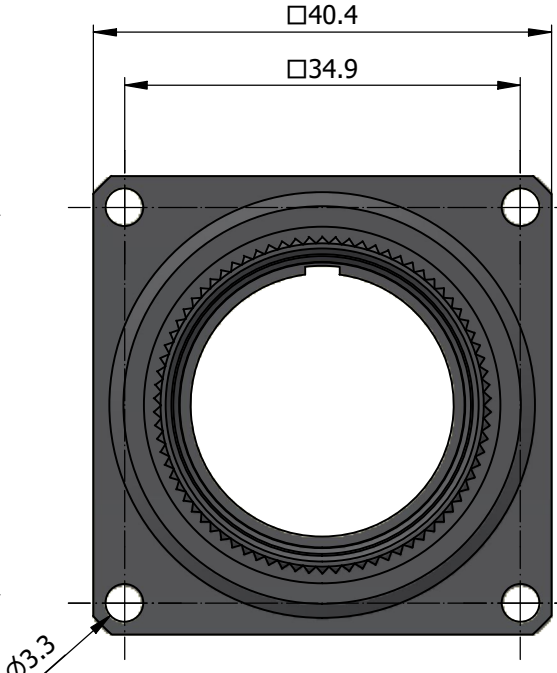
1) Shell Dimensions 1
