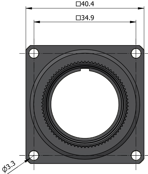
1) Shell Dimensions 1)
